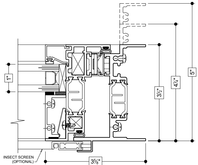
31 RIGHT JAMB - OFFSET (PROJECT-IN)
