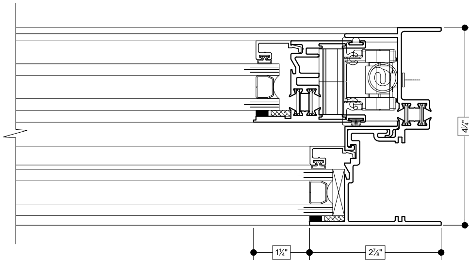
4 RIGHT JAMB (SINGLE HUNG)
