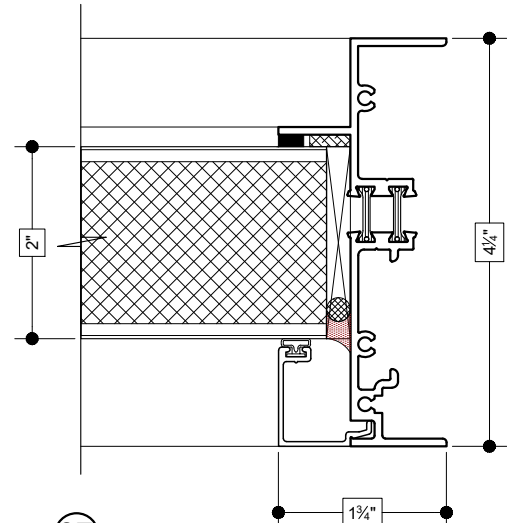
37 RIGHT JAMB (FIXED PANEL)
