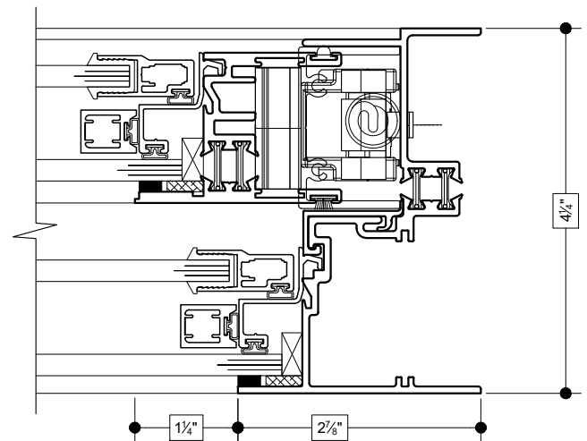
17 RIGHT JAMB (SINGLE HUNG)
