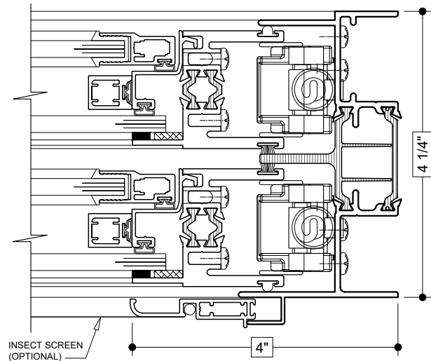
8 RIGHT JAMB (DOUBLE HUNG)
