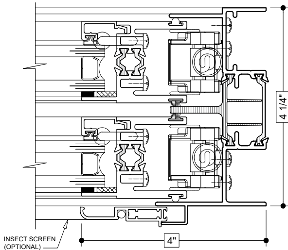
7 RIGHT JAMB (DOUBLE HUNG)
