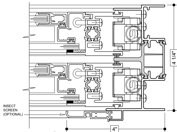
10 RIGHT JAMB (DOUBLE HUNG)
