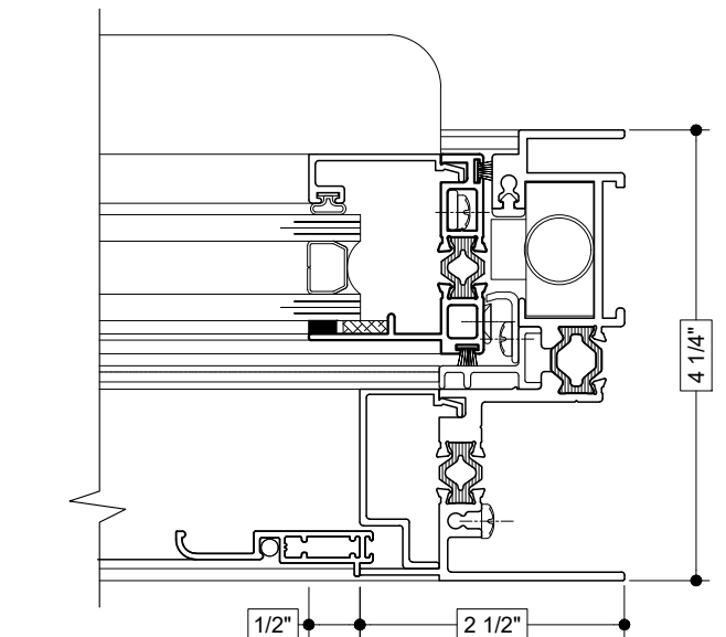
24 RIGHT JAMB (SINGLE HUNG)
