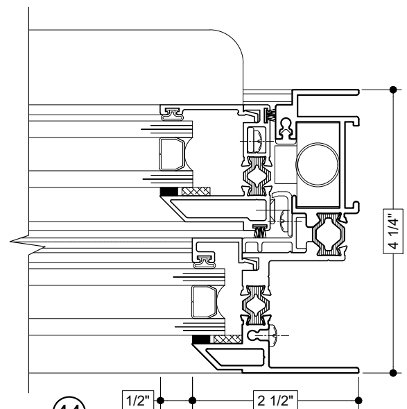
44 RIGHT JAMB (SINGLE HUNG)
