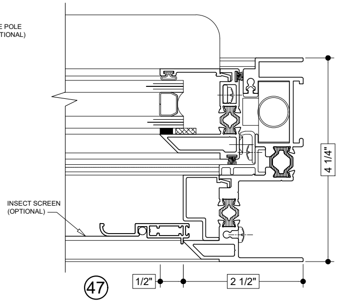
RIGHT JAMB (SINGLE HUNG)
