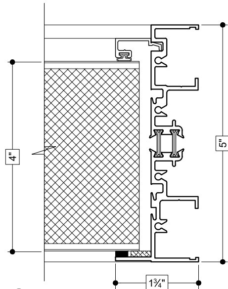
23 RIGHT JAMB (FIXED PANEL)
