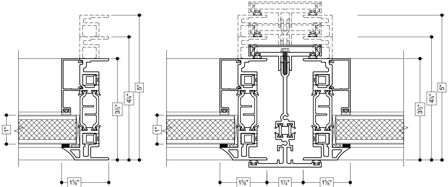
RIGHT JAMB (FIXED PANEL)
