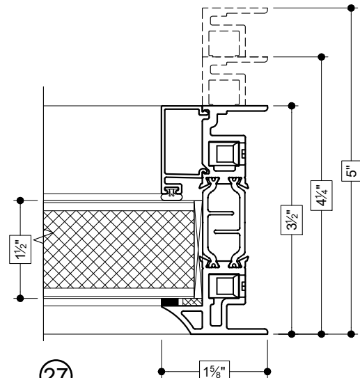
27 RIGHT JAMB (FIXED PANEL)
