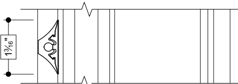
2 PIECE EXTERIOR MUNTIN (CONCAVE)
