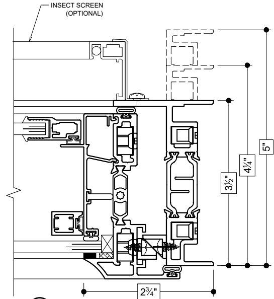
42 RIGHT JAMB (OUTSWING)
