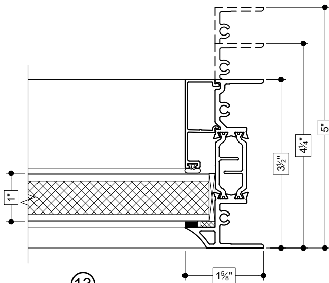
13 RIGHT JAMB (FIXED PANEL)
