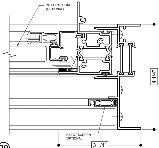
20 RIGHT JAMB
